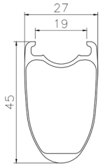
PERFIL DELANTERO / TRASERO
