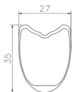
PERFIL DELANTERO / TRASERO
